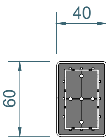
Bottom Plan 1:3
