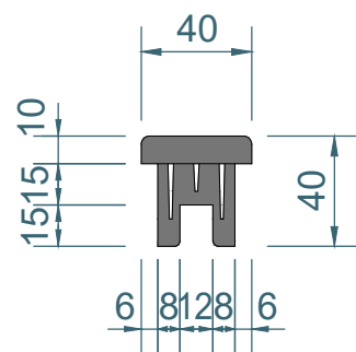
Elevation 1:3
