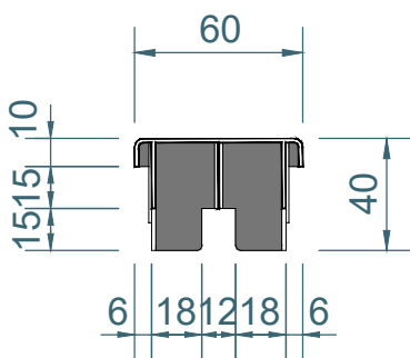
a-a Section 1:3
