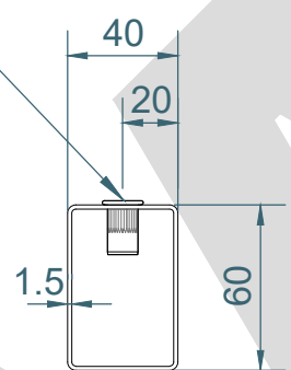
2-2 Section 1:3
