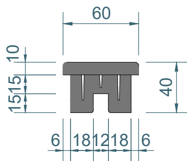
Side Elevation 1:3
